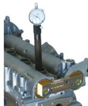
Anwendungsbild (Satz ohne Messuhr)
