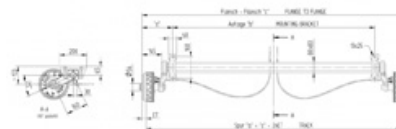
Abmessungen
