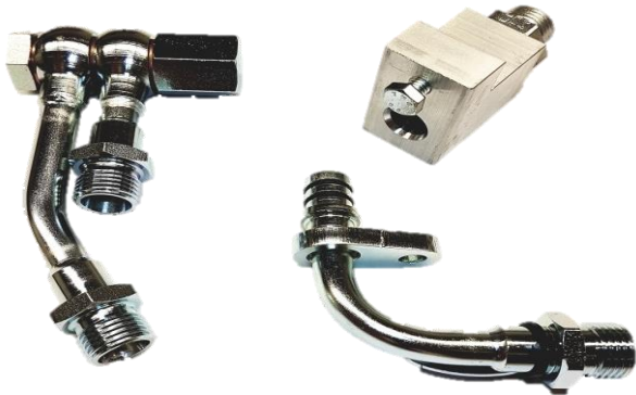
Adapter 400.433.000 Anschluss zwischen Ölkühlerleitung und Getriebe
