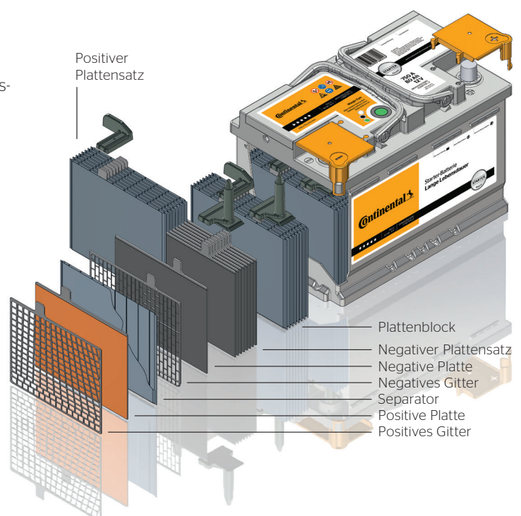
Blei-Säure-Technologie: Batterieaufbau
