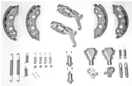
Radbremseninnenteile verpackt
